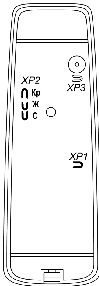
Рисунок 2. Расположение трех переключателей «номер считывателя» (XP2), переключателя «отключение концевого резистора» (XP1) и «тип выходного интерфейса» (XP3)
