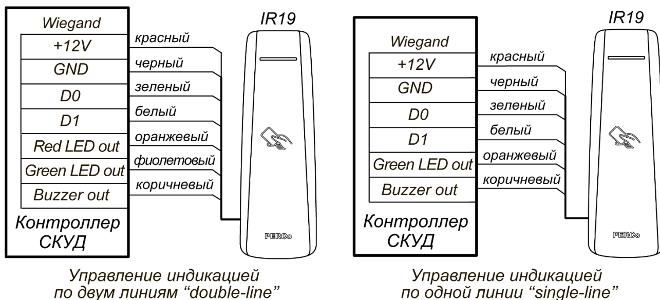
Рисунок 4. Схема подключения считывателя к внешним устройствам с использованием интерфейса Wiegand
