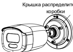
Рисунок 2-12 Установка распределительной коробки
